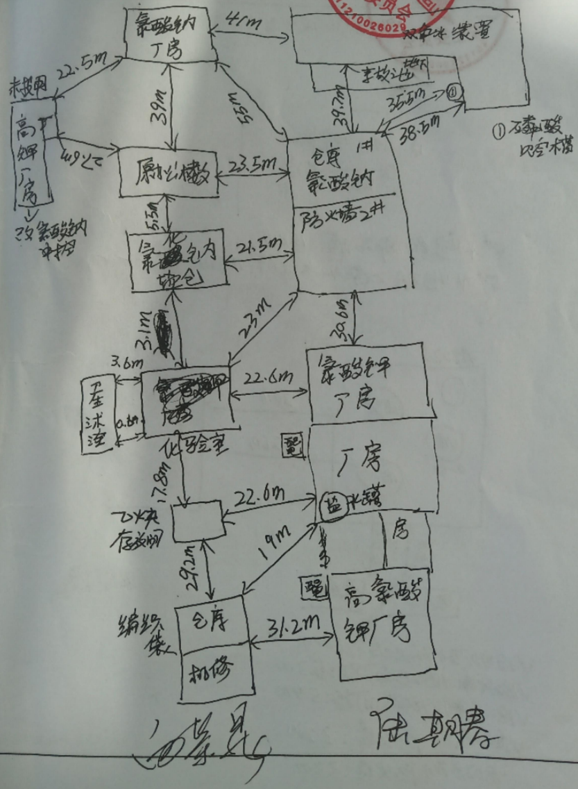
生产区域平面布置示意图
